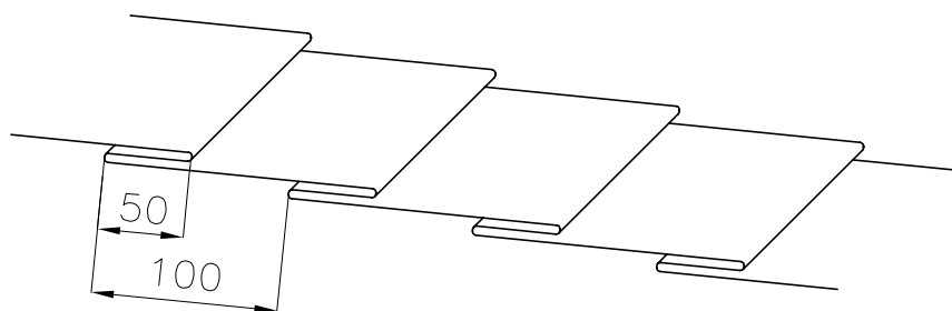
折込構造図
