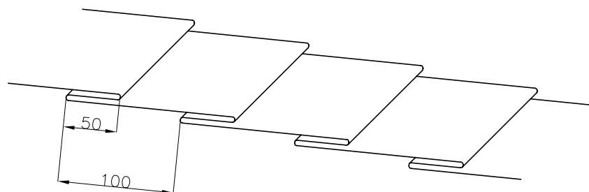
折込構造図
