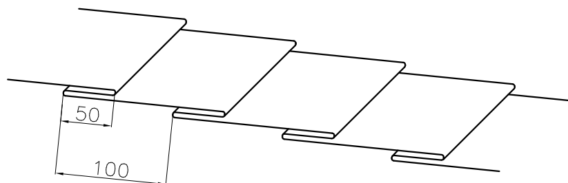
折込構造図
