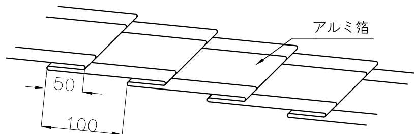
折込構造図
