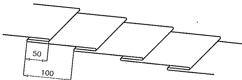
折込構造図
