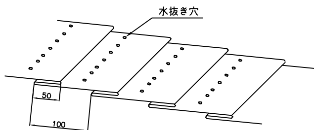
折込構造図
