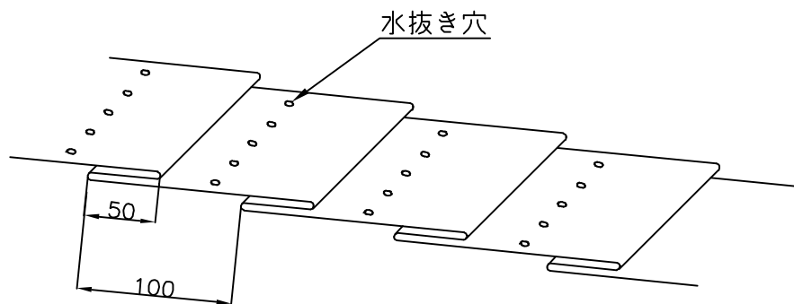
折込構造図
