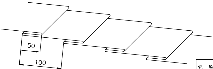
折込構造図
