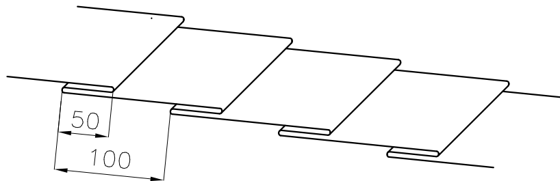
折込構造図
