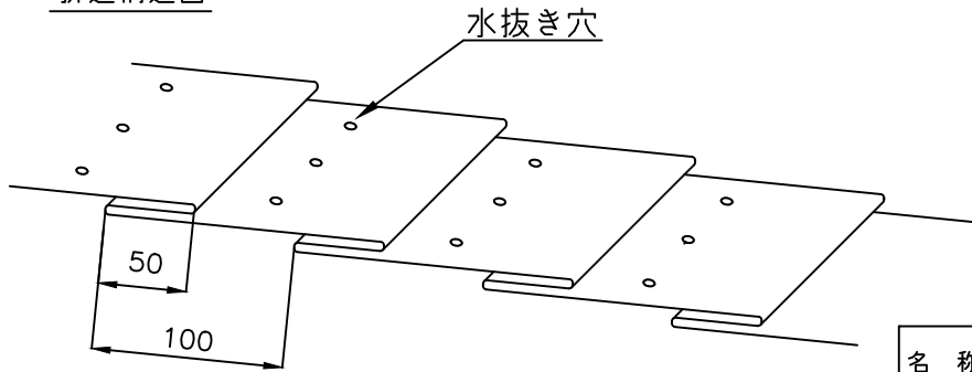
折込構造図
