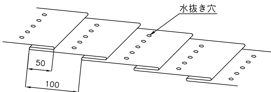
折込構造図
