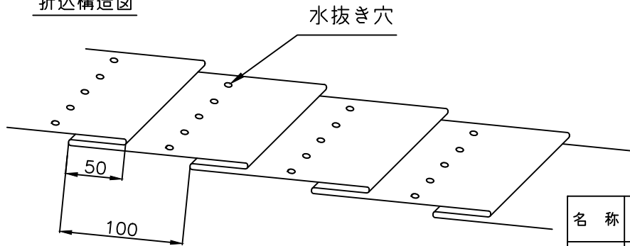
折込構造図
